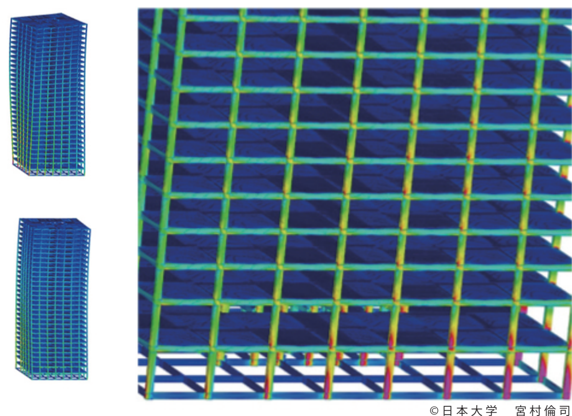
図1. 超高層ビルの地震応答シミュレーション。建物全体の变形（変形は30倍）。色はひずみの度合いを示している。
