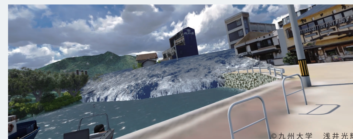
図5. 先端的三次元の津波シミュレーション
